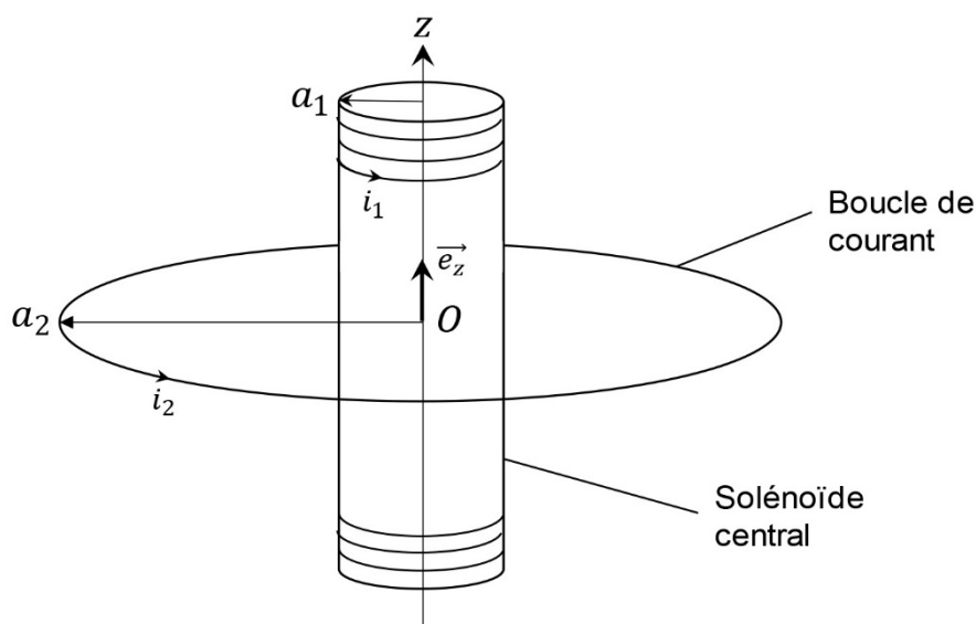
Figure 7 - Représentation schématique du système solénoïde central – plasma dans le tokamak
