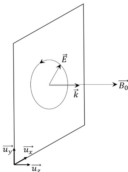
Figure 9 - Onde de polarisation circulaire gauche se propageant parallèlement au champ magnétique \vec{B}_0
