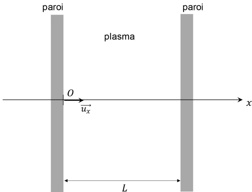
Figure 4 - Géométrie de l'enceinte contenant le plasma
