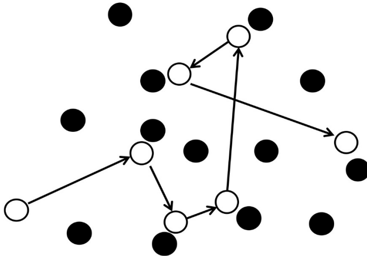
Figure 5 - Marche au hasard : la boule blanche représente l'entité diffusante, les boules noires les autres entités du milieu avec lesquelles elle est susceptible de rentrer en collision
