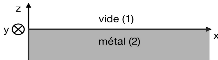
FIGURE 2 – Schéma de l'interface vide-métal.
