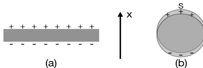
FIGURE 1 – Illustration des oscillations de charge à la surface d'une plaque mince (a) et d'une sphère ou d'un cylindre (b).
