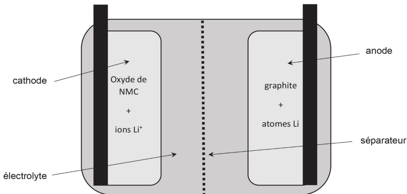
Figure 10 - Schéma d'une cellule Li ion
