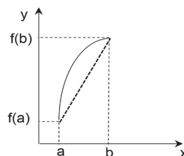
Figure 13 - Méthode des trapèzes
