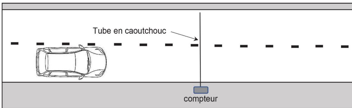
Figure 1 - Capteur pneumatique
