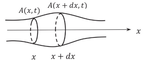
Figure 3 - Système étudié : tranche d'air d'épaisseur dx
