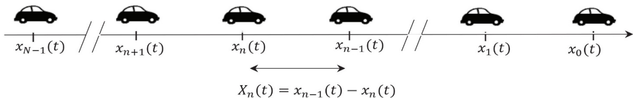
Figure 6 - Schéma du problème
