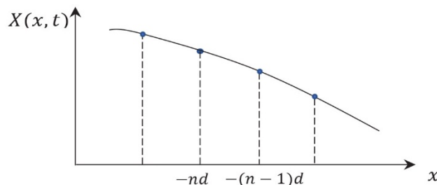
Figure 8 - Représentation de X(x, t) à t fixé
