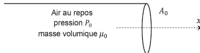
Figure 2 - Tube de section A_0 rempli d'air au repos
