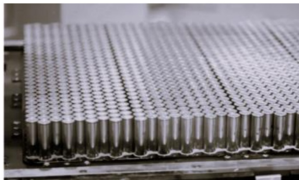
Figure 9 - Batterie de la Tesla model 3
