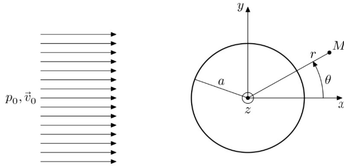
Figure 11 Modélisation de l'écoulement de l'air autour du cylindre
