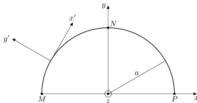
Figure 15 Profil et repère cartésien local (x', y')
