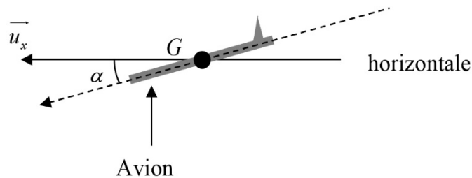
Figure 6 - Avion en mouvement rectiligne uniforme sans propulsion
