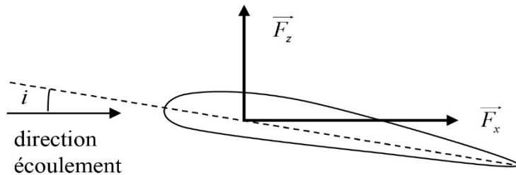
Figure 4 - Décomposition des efforts aérodynamiques : portance et traînée
