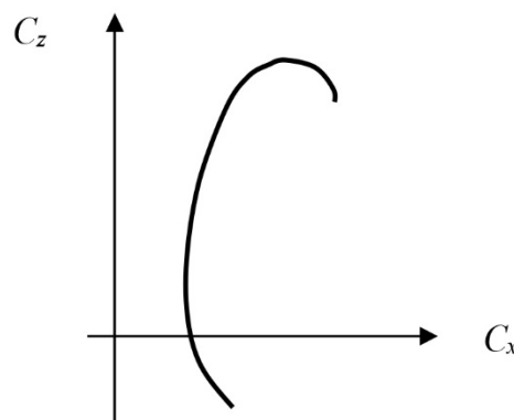
Figure 7 - Polaire d'une aile
