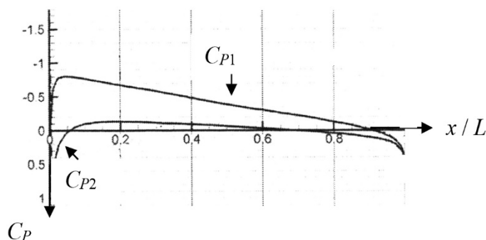
Figure 3 - Coefficient de pression sur l'intrados et l'extrados
