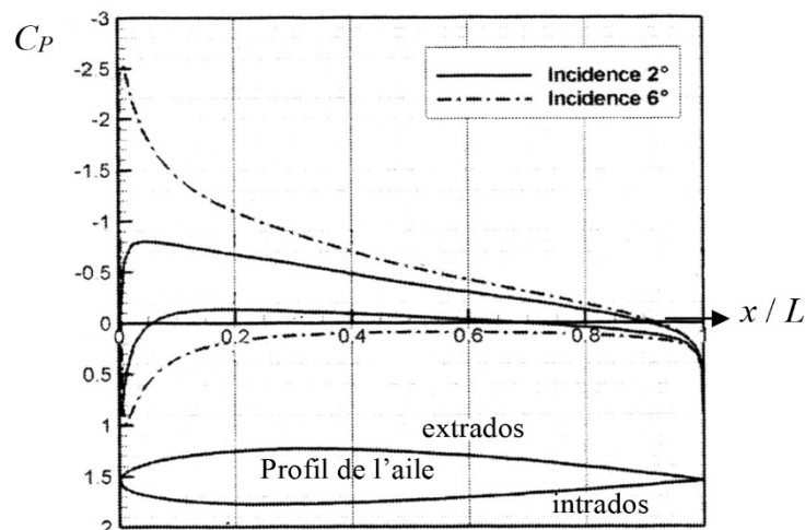
Figure 5 - Influence de l'incidence sur le C_P
