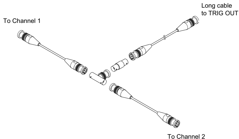
Figure 48 Câble d'étalonnage utilisateur pour un oscilloscope à deux voies
