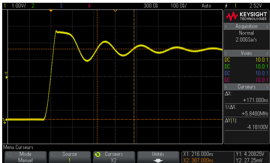
Figure 41 Mesure par curseurs de la fréquence des oscillations transitoires de l'impulsion
