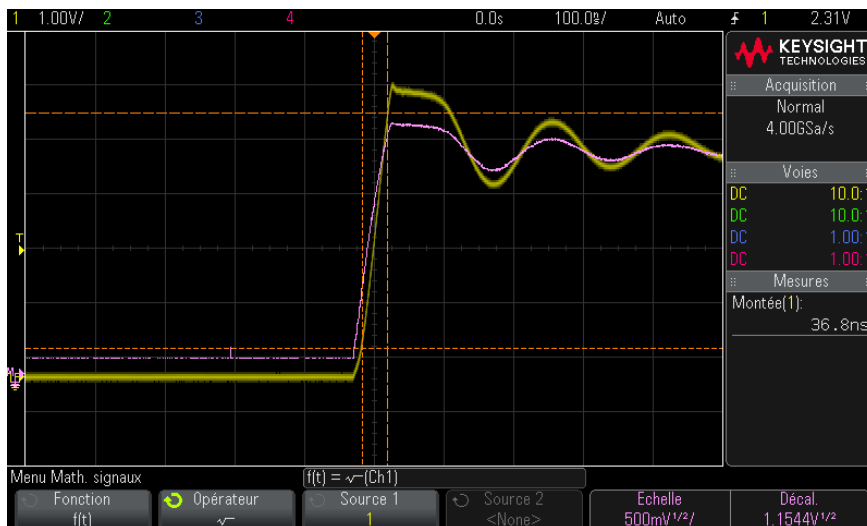
Figure 10 Exemple de fonction \sqrt{\phantom{x}} (Racine carrée)
