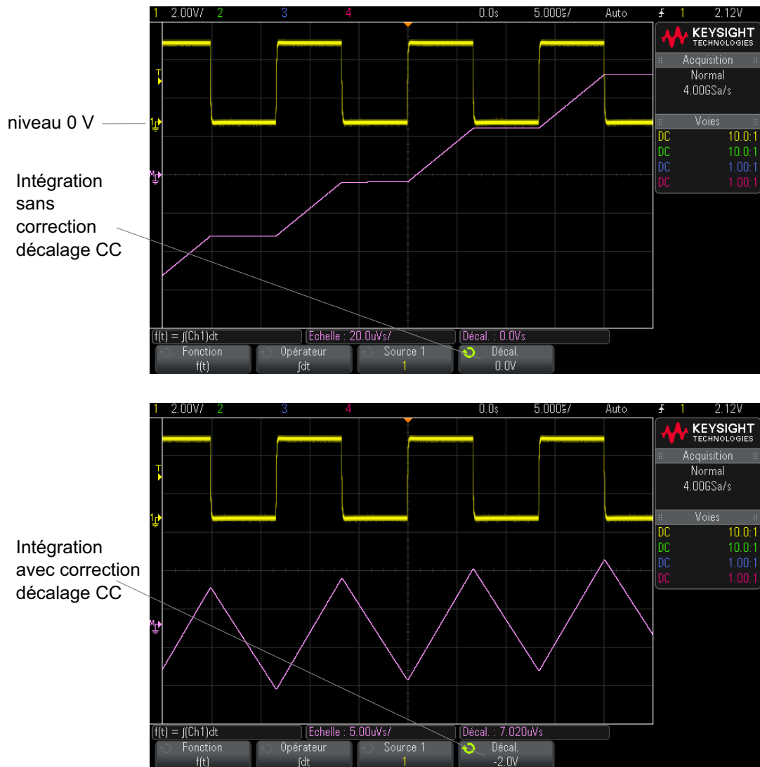
Figure 8 Intégration et décalage du signal
