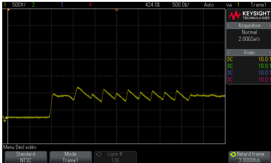
Figure 32 Utilisation du retard de trame pour synchroniser sur la trame de couleur 1 ou 3 (mode Trame 1)
