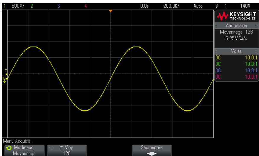
Figure 39 128 moyennes utilisées pour réduire le bruit aléatoire
