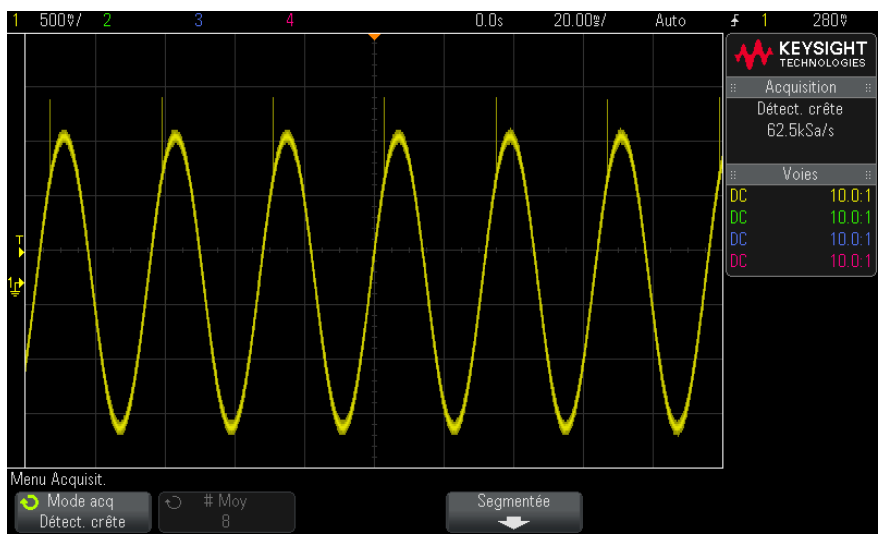
Figure 37 Sinusoïde avec impulsion transitoire, mode de détection de crête
