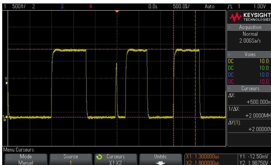
Figure 44 Déplacement simultané des curseurs pour rechercher des variations de largeur d'impulsion
