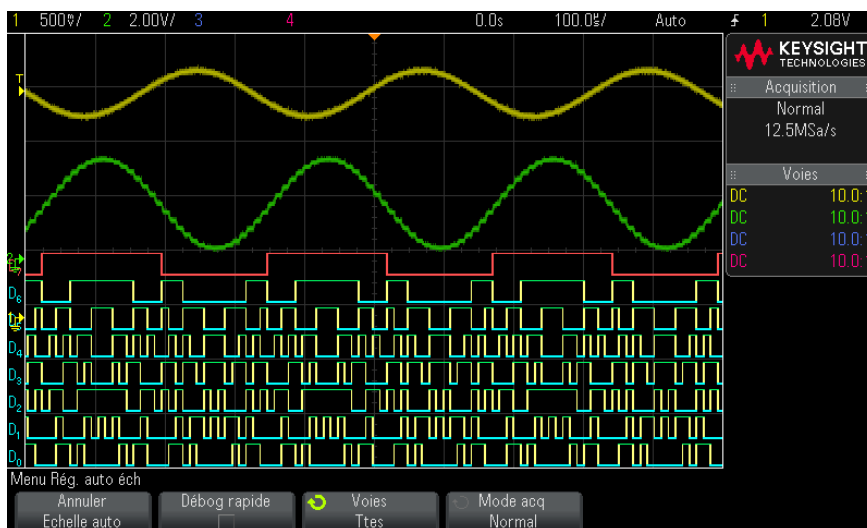
Figure 20 Exemple : réglage d'échelle automatique des voies numériques (modèles MSO uniquement)
