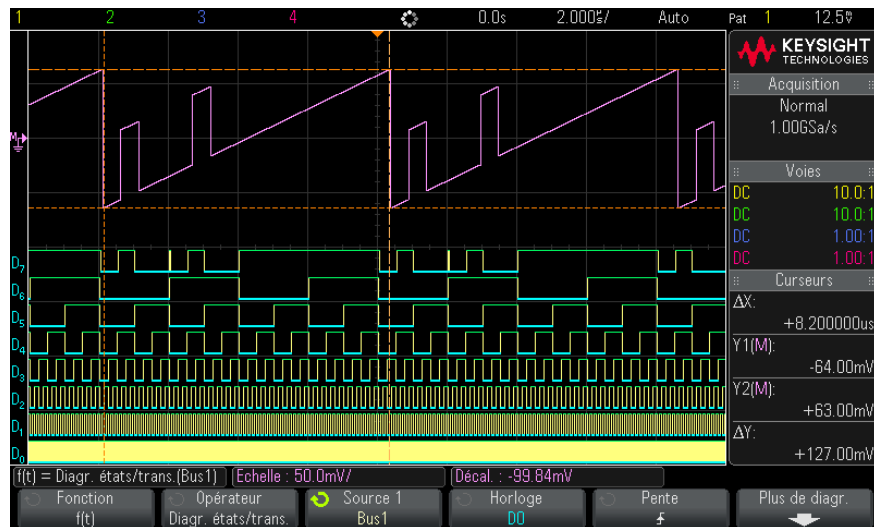
Figure 19 Exemple de diagramme d'état du bus logique
