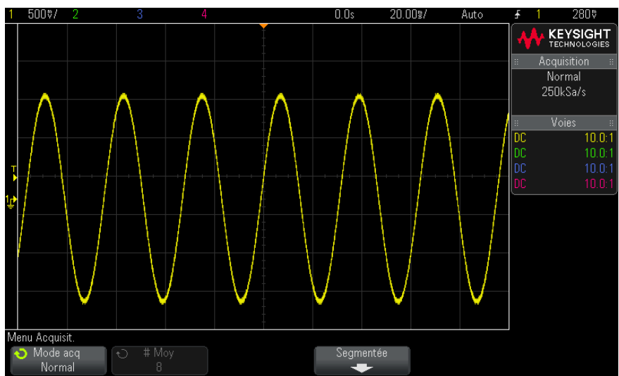
Figure 36 Sinusoïde avec impulsion transitoire, mode Normal
