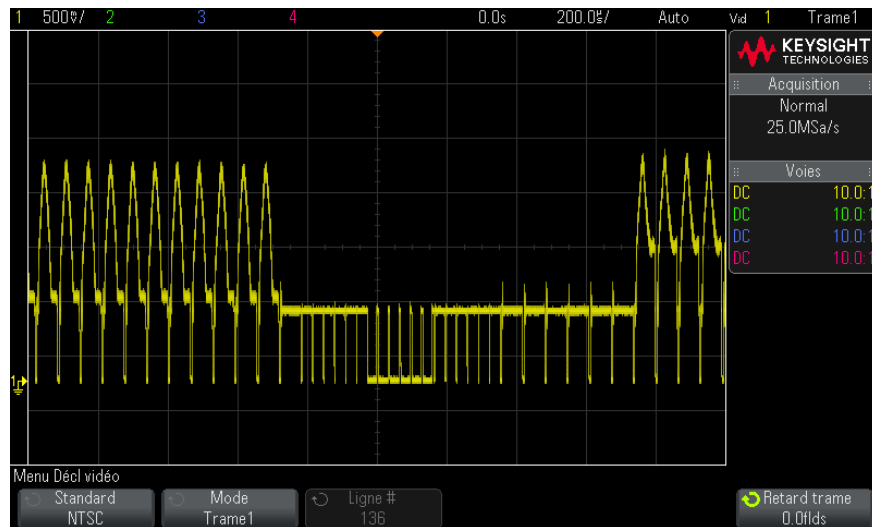
Figure 29 Déclenchement sur la trame 1
