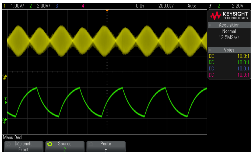
Figure 26 Modulation d'amplitude représentée à une intensité de 40%
