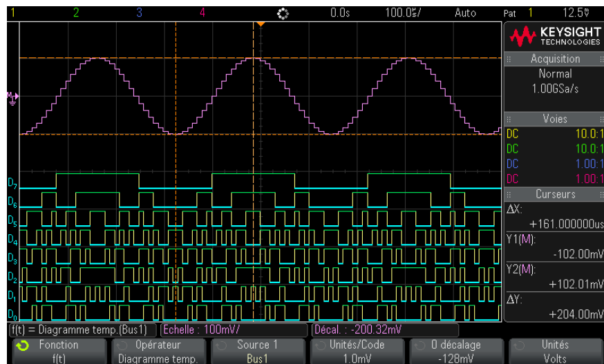
Figure 18 Exemple de diagramme de temporisation du bus logique
