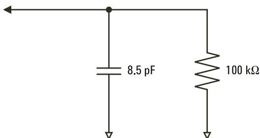
Figure 21 Circuit équivalent de sonde basse fréquence et CC
