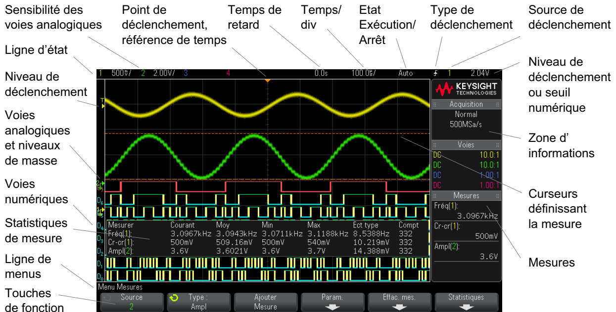
Figure 1 Interprétation de l'affichage de l'oscilloscope
