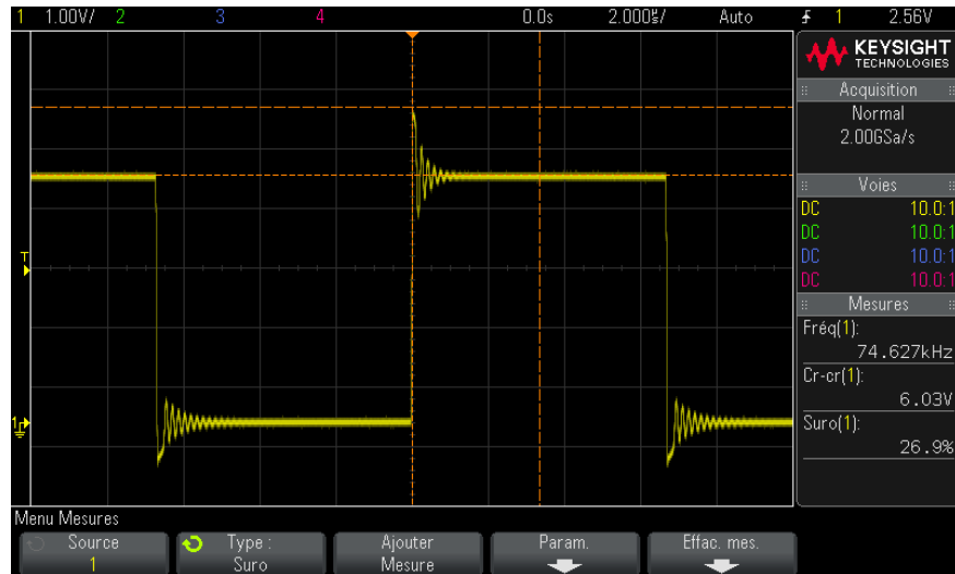
Figure 46 Mesure automatique de la suroscillation
