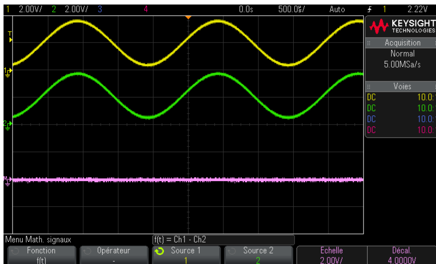
Figure 5 Exemple de soustraction de la voie 2 de la voie 1
