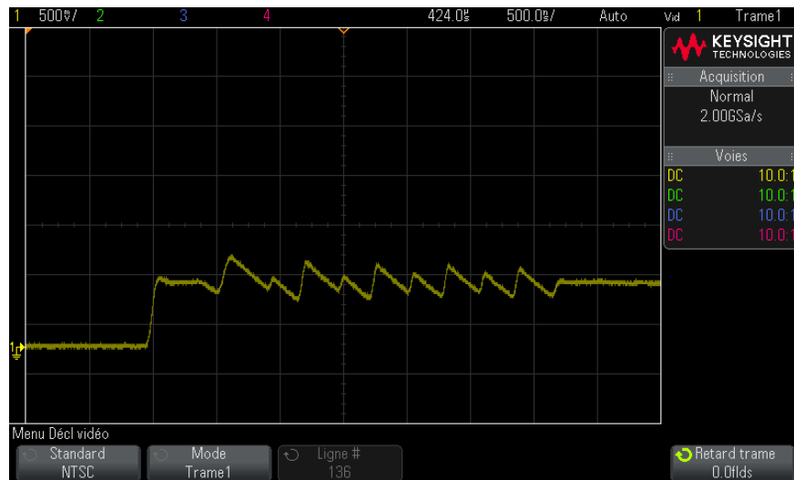
Figure 31 Déclenchement sur la trame de couleur 1 en alternance avec la trame de couleur 3
