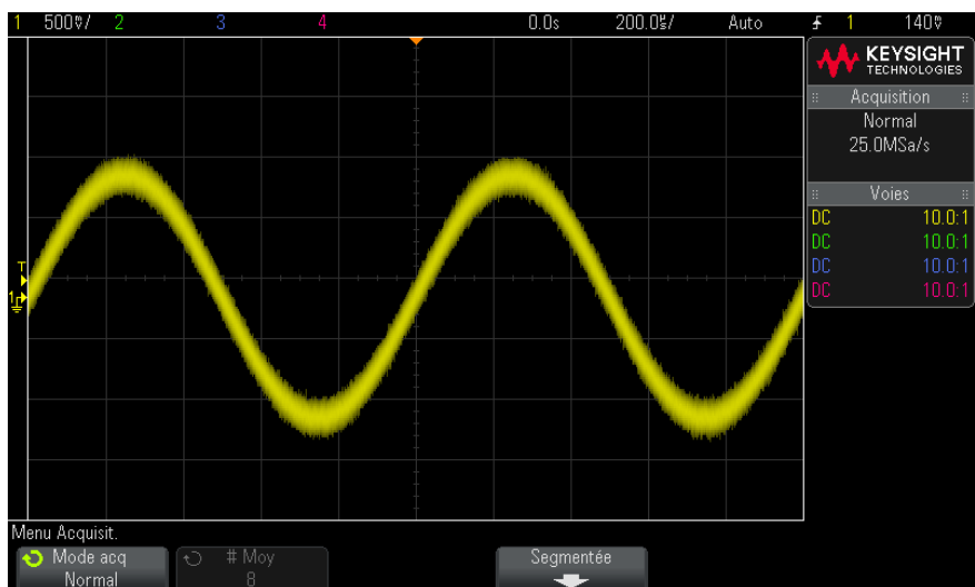
Figure 38 Bruit aléatoire sur le signal affiché
