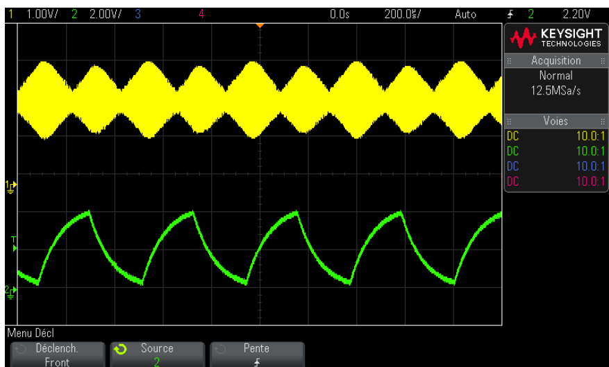
Figure 25 Modulation d'amplitude représentée à une intensité de 100%
