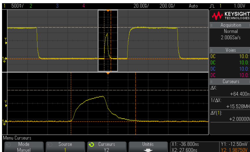
Figure 42 Curseurs de suivi - Fenêtre de zoom
