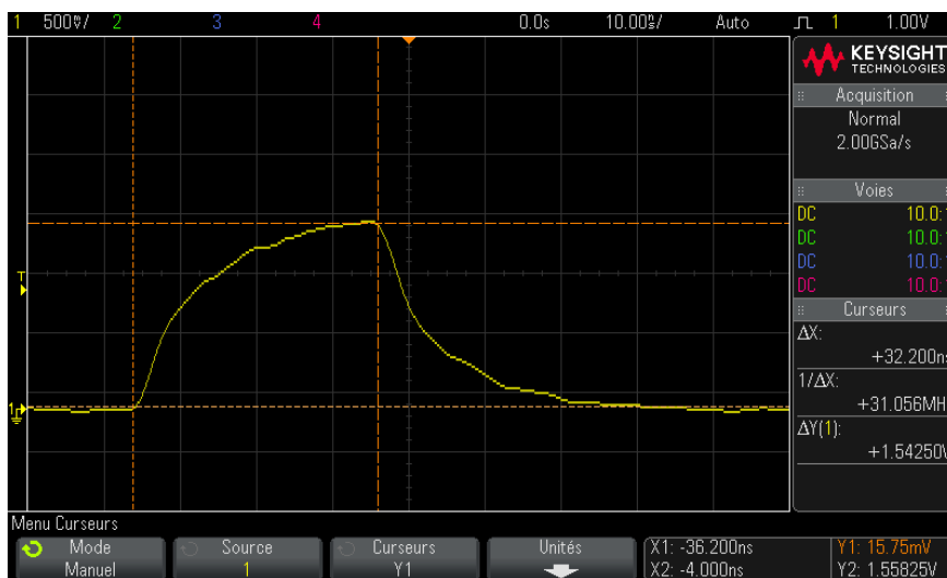
Figure 40 Curseurs utilisés pour mesurer des largeurs d'impulsion (autres que les points de seuil à mi-hauteur)
