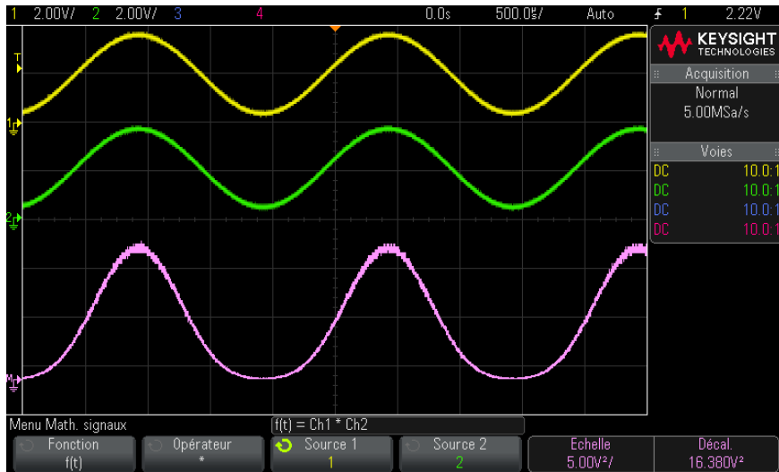
Figure 6 Exemple de multiplication de la voie 1 par la voie 2
