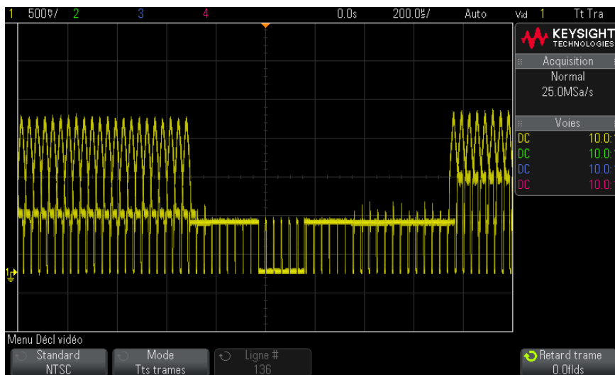
Figure 30 Déclenchement sur toutes les trames
