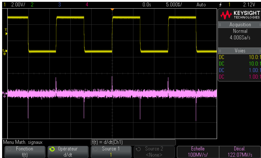
Figure 7 Exemple de fonction Dérivation
